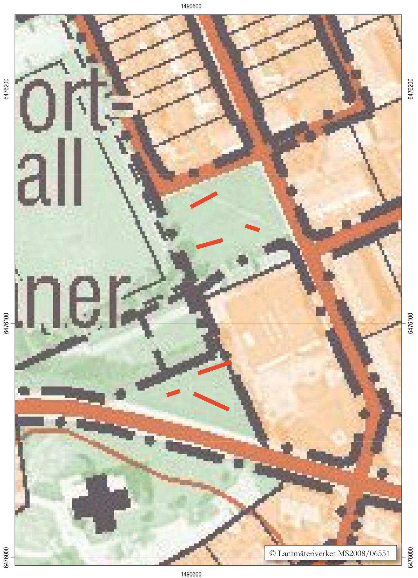
Figur 3. Utdrag ur digitala Fastighetskartan med schakten markerade. Skala 1:1000.
